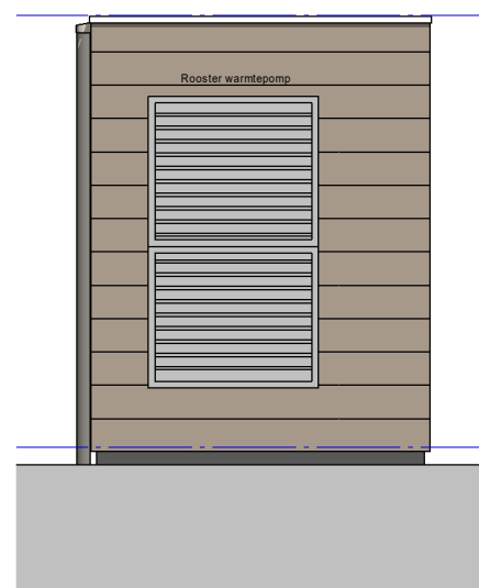
linkergevel
